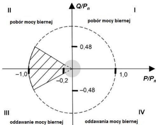
Rys. 2. Zdolność do generacji mocy biernej w obciążeniowym układzie
